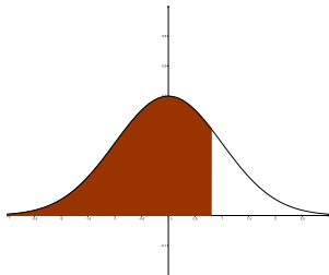
FIGURE : Loi normale : \Phi(0,6) est l'aire de la partie colorée
