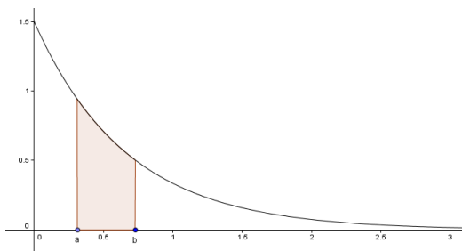
FIGURE : Densité de la loi exponentielle de paramètre \lambda = 1,5 avec P(a \leq X \leq b) .
