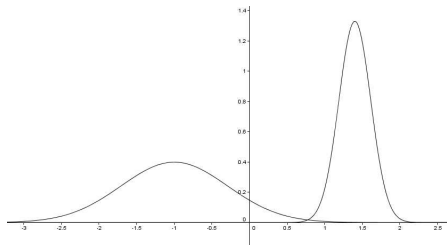
FIGURE : Densités de lois normales : à gauche \mathcal{N}(-1; 1) et à droite \mathcal{N}(1,4; 0,09)
