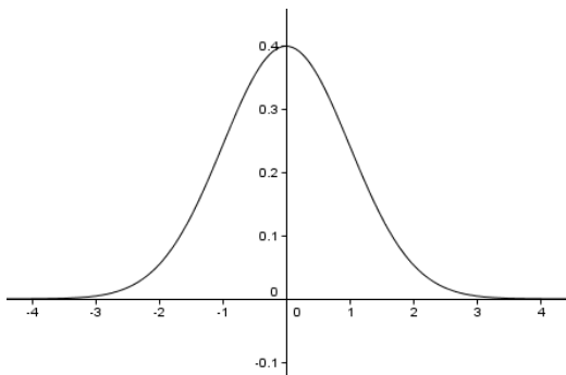
FIGURE : Densité de la loi normale centrée réduite
