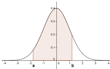
FIGURE : P(a \leq X \leq b) est l'aire de la partie colorée
